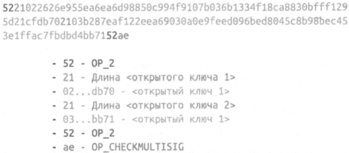
Рис. 8.20. Сценарий RedeemScript для p2sh
