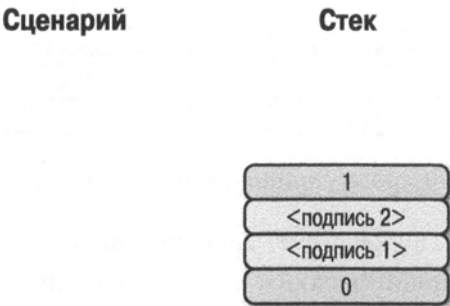
Рис. 8.19. Конечное состояние сценария p2sh, если он вычислялся программным обеспечением, разработанным до появления протокола BIP0016
