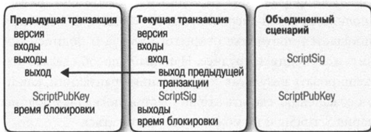
Рис. 7.3. Объединение сценариев ScriptPubKey и ScriptSig
