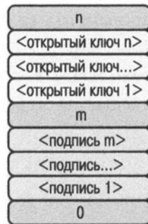
Рис. 8.7. Третья стадия выполнения простой мультиподписи
