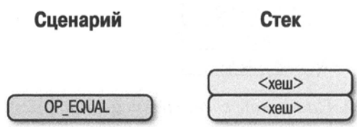
Рис. 13.15. Третья стадия выполнения сценария p2sh-p2wpkh
