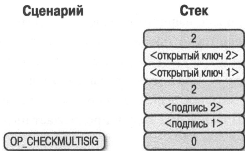
Рис. 8.22. Пятая стадия выполнения сценария p2sh
