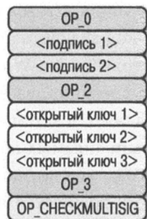
Рис. 13.28. Третья стадия выполнения сценария r2wrkh
