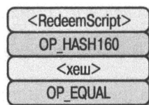
Рис. 8.14. Последовательность команд для p2sh, выполняющая особое правило
