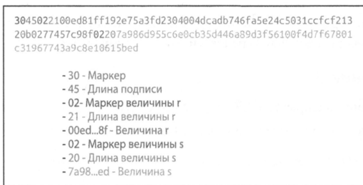
Рис. 4.4. Формат DER
