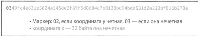
Рис. 4.3. Сжатый формат SEC
