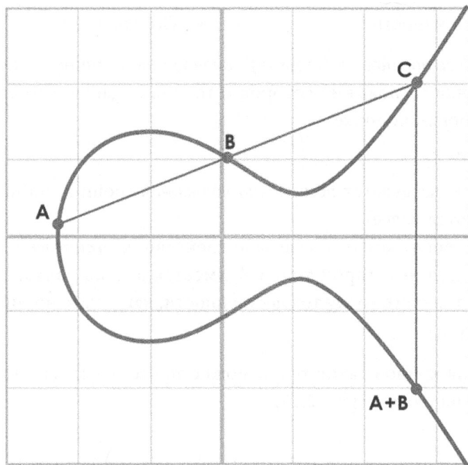
Рис. 2.14. Сложение точек
