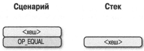
Рис. 13.14. Вторая стадия выполнения сценария p2sh-p2wpkh
