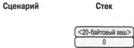
Рис. 13.17. Пятая стадия выполнения сценария p2sh-p2wprkh
