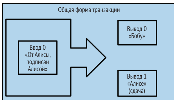
Рис. 2.5 ❖ Наиболее общая форма транзакции
