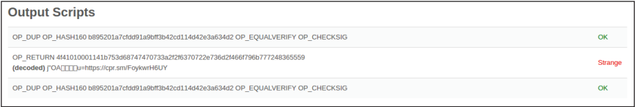
Рис. 12.3 ❖ Скрипты в эмиссионной транзакции
