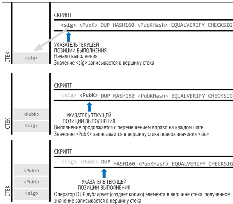
Рис. 6.5 ❖ Выполнение скрипта для транзакции типа P2PKH (часть 1 из 2)
