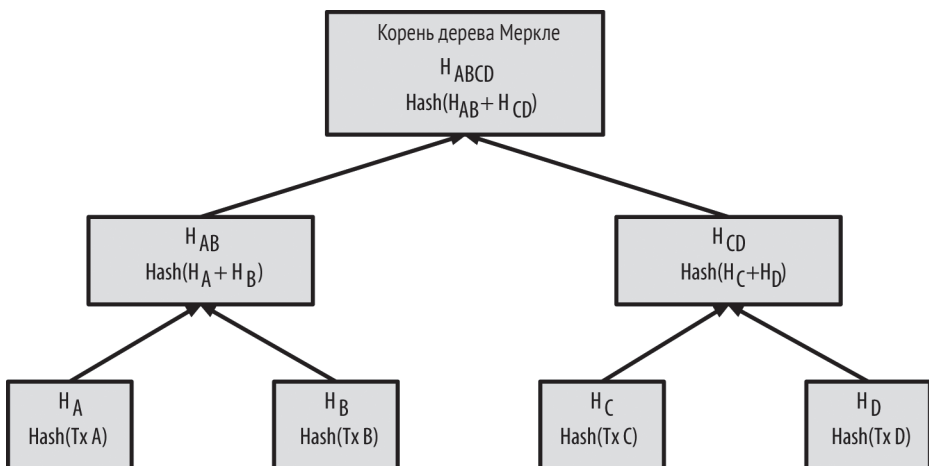
Рис. 9.2 ❖ Вычисление хэш-значений узлов в дереве Меркле
