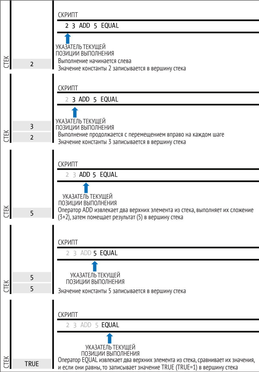
Рис. 6.4 ❖ Скрипт проверки биткойн-транзакции, вычисляющий простое арифметическое выражение
