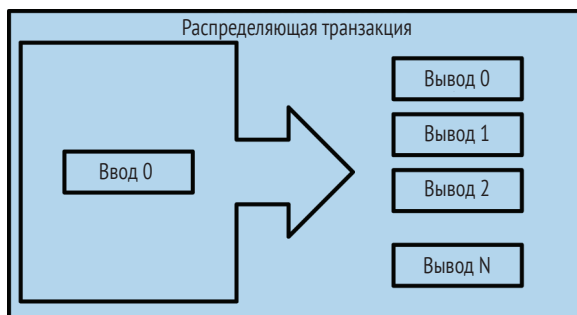
Рис. 2.7 ❖ Транзакция, распределяющая денежные средства
