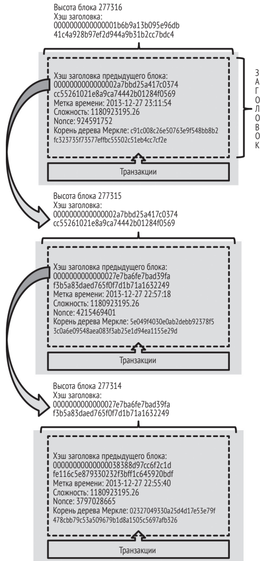
Рис. 9.1 ❖ Блоки, связанные в цепочку с помощью ссылки на хэш-значение заголовка предыдущего блока
