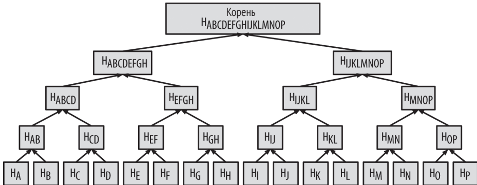
Рис. 9.4 ❖ Дерево Меркле, объединяющее большое количество элементов данных
