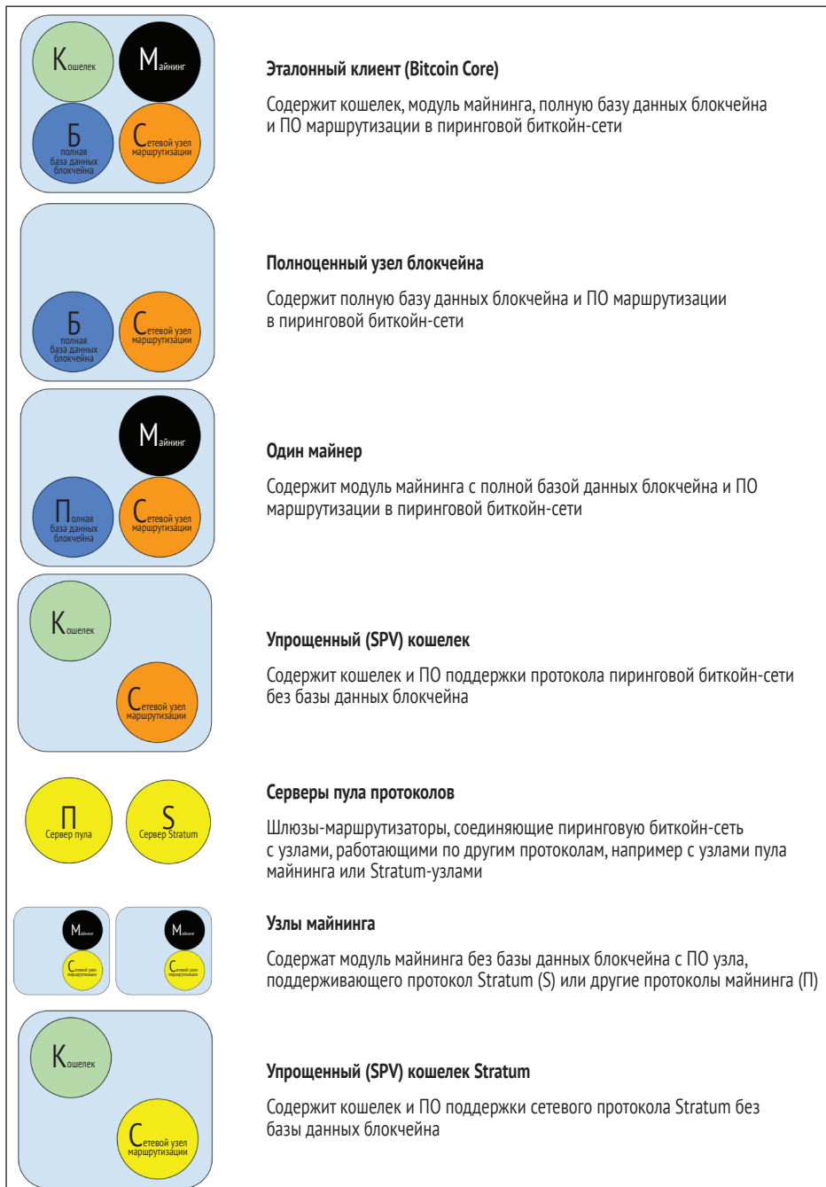
Рис. 8.2 ❖ Различные типы узлов в расширенной биткойн-сети
