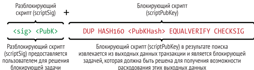
Рис. 6.3 ❖ Объединение scriptSig и scriptPubKey для выполнения проверочного скрипта транзакции
