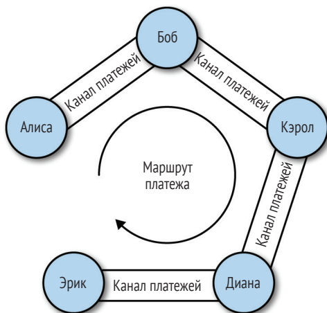
Рис. 12.9 ❖ Последовательность двунаправленных каналов платежей, связанных в сеть Lightning Network, которая может обеспечить маршрутизацию платежа от Алисы к Эрику
