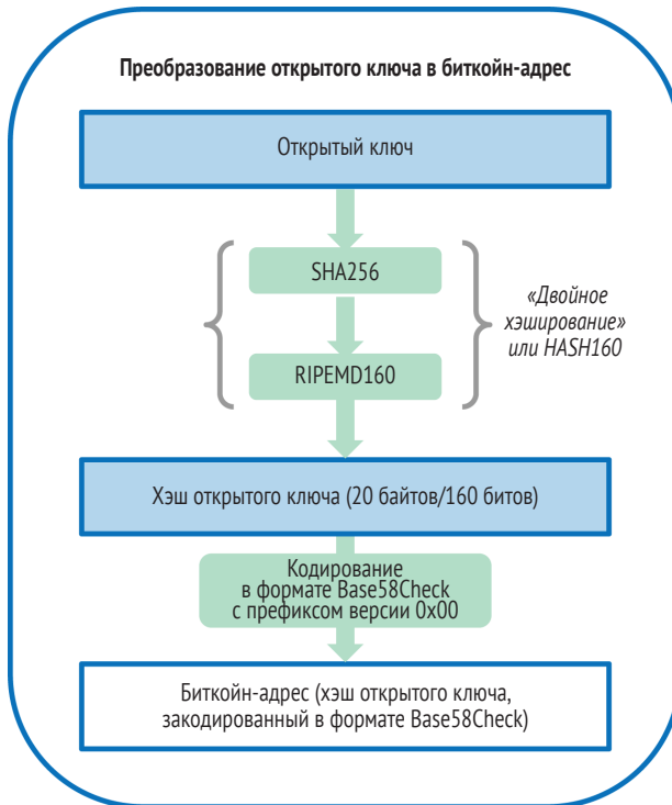
Рис. 4.5 ❖ Схема преобразования открытого ключа в биткойн-адрес
