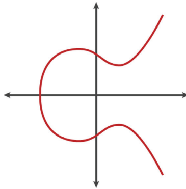
Рис. 4.2 ❖ Эллиптическая кривая
