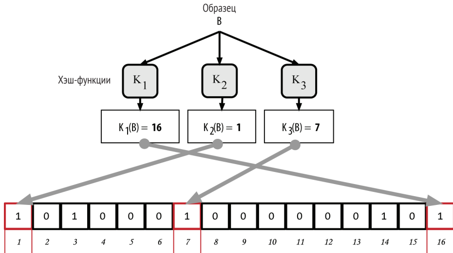
Рис. 8.10 ❖ Добавление второго шаблона «В» в простой фильтр Блума
