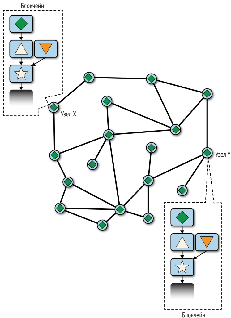
Рис. 10.6 ❖ Наблюдение за событиями разветвления цепочки блокчейна: вся сеть переходит на новую самую длинную цепочку
