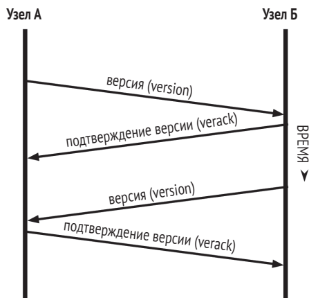
Рис. 8.4 ❖ Начальная процедура «рукопожатия» между партнерами
