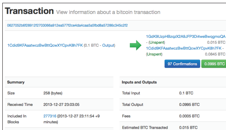
Рис. 2.8 ❖ Транзакция Алисы, выполняющая оплату в кафе Боба
