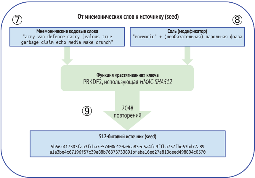
Рис. 5.7 ❖ От мнемонического кода к источнику
