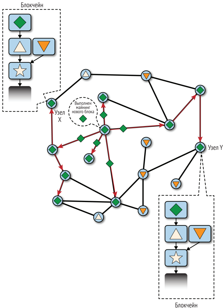
Рис. 10.5 ❖ Наблюдение за событиями разветвления цепочки блокчейна: новый блок наращивает одну из ветвей, заставляя сеть пересмотреть статус соответствующей цепочки
