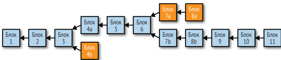
Рис. 10.9 ❖ Цепочка блокчейна с разветвлениями
