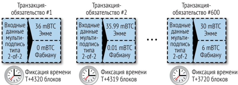
Рис. 12.7 ❖ Для каждой очередной транзакции-обязательства устанавливается более короткий срок блокировки по времени, позволяя расходовать ее раньше, чем предыдущие обязательства станут валидными
