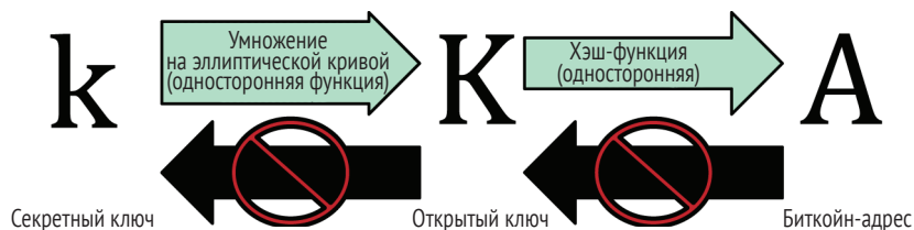
Рис. 4.1 ❖ Секретный ключ, открытый ключ и биткойн-адрес
