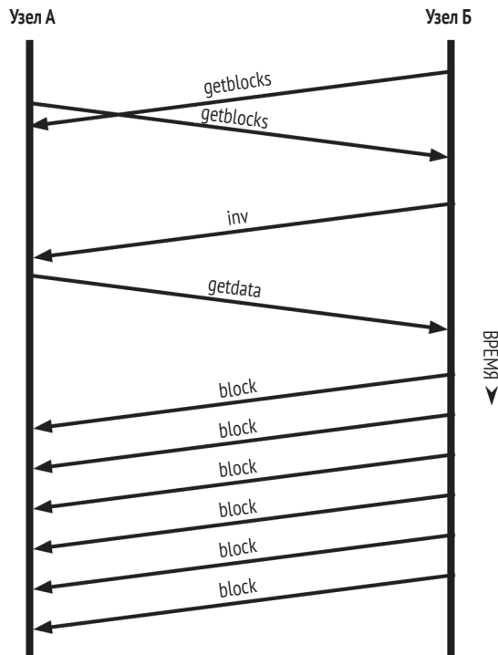
Рис. 8.6 ❖ Узел синхронизирует структуру данных блокчейна, получая недостающие блоки от партнера
