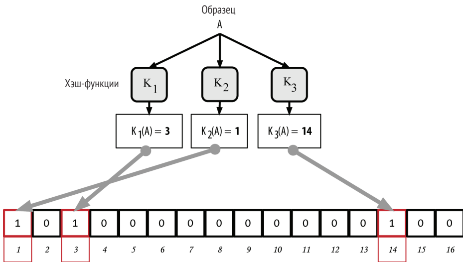
Рис. 8.9 ❖ Добавление шаблона «А» в простой фильтр Блума
